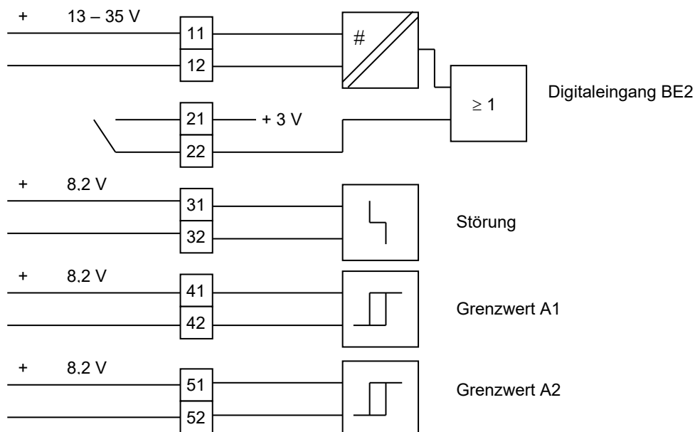
Bild 7 Elektrischer Anschluss Binär-Modul / Digital I/O Module
