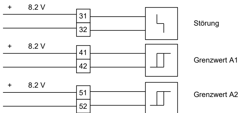
Bild 8 Elektrischer Anschluss Schlitzinitiatoren-Modul / Inductive Limit Switches
