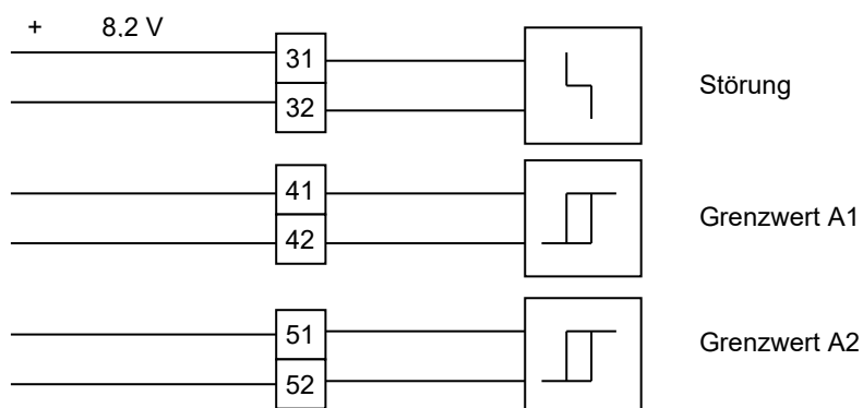
Bild 9 Elektrischer Anschluss Kontakt-Modul / Mechanic Limit Switches
