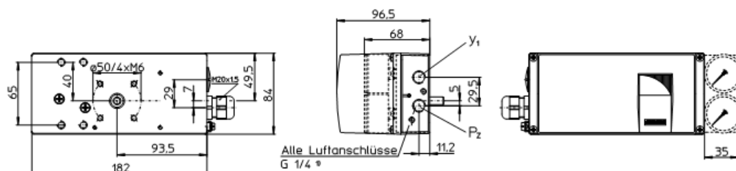
Bild 1 Metallgehäuse Standard
