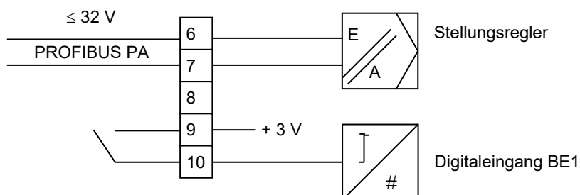
Bild 4 Elektrischer Anschluss Grundgerät PROFIBUS PA
