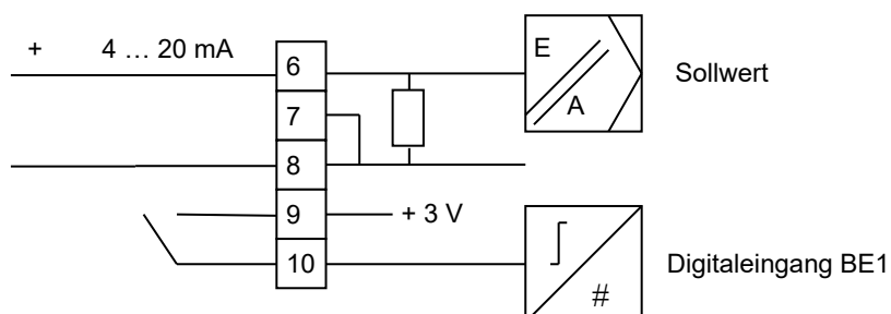
Bild 3 Elektrischer Anschluss Grundgerät 2 Leiter
