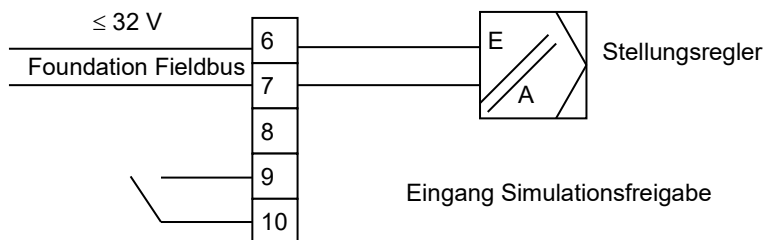
Bild 5 Elektrischer Anschluss Grundgerät Foundation Fieldbus
